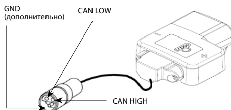
GND (дополнительно) CAN LOW CAN HIGH
